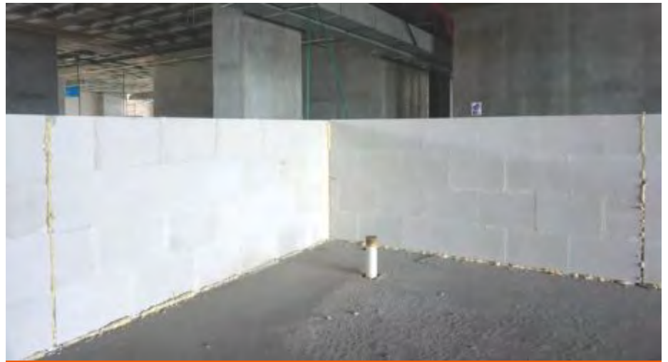
Fig. 7: Junta de control a cada 15 m 2 de muro.
